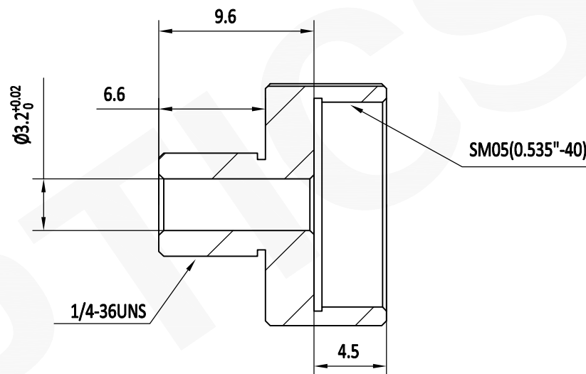
剖面E-E
