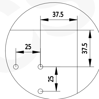
局部视图A 比例1:2
