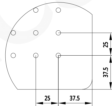
局部视图A 比例1:2
