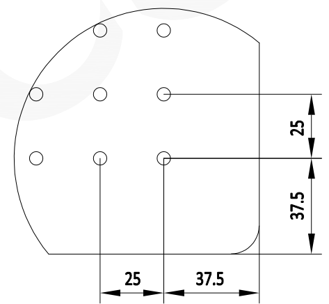
局部视图A 比例1:2
